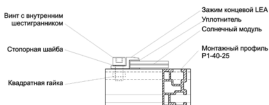
Начальное и конечное крепление аморфных модулей
