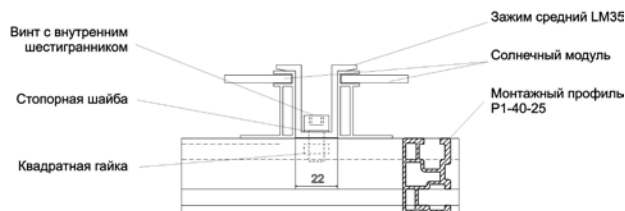
Среднее крепление аморфных модулей
