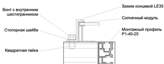
Начальное и конечное крепление аморфных модулей
